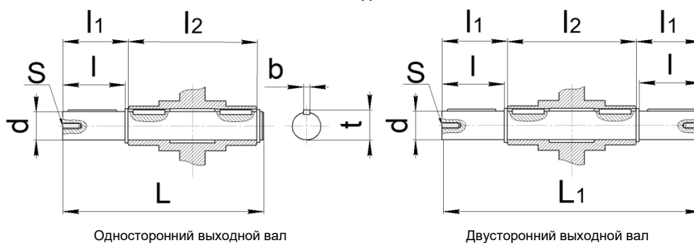
Односторонний выходной вал
