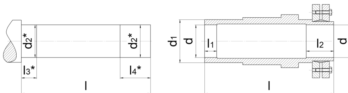
РАЗМЕРЫ ПОЛОГО ГЛАДКОГО ВЫХОДНОГО ВАЛА СО СТЯЖНОЙ МУФТОЙ КН, КНФ, КНЗ
