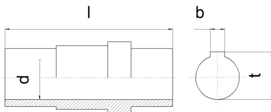
РАЗМЕРЫ ПОЛОГО ВЫХОДНОГО ВАЛА СО ШПОНОЧНЫМ ПАЗОМ КА, KAF, KAZ
