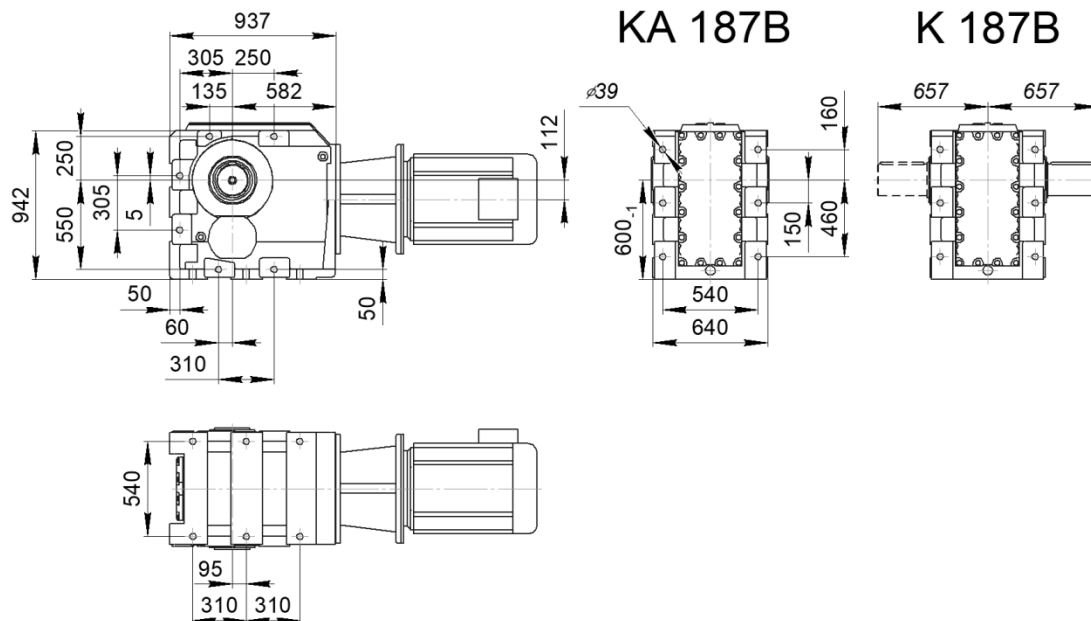
ГАБАРИТНЫЕ И ПРИСОЕДИНИТЕЛЬНЫЕ РАЗМЕРЫ РЕДУКТОРА КА 187В, К 187В
