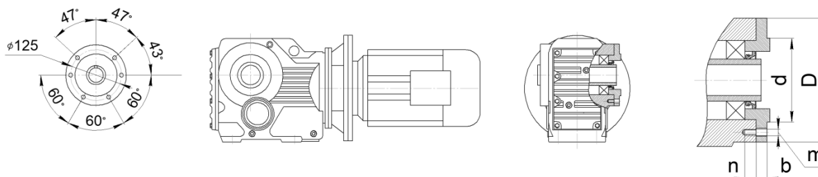
РАЗМЕРЫ ВЫХОДНОГО ФЛАНЦА РЕДУКТОРА KAZ, KVZ
