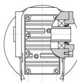
РАЗМЕРЫ ВЫХОДНОГО ФЛАНЦА РЕДУКТОРА KAZ, KVZ
