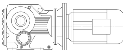
РАЗМЕРЫ ВЫХОДНОГО ФЛАНЦА РЕДУКТОРА KAZ, KVZ
