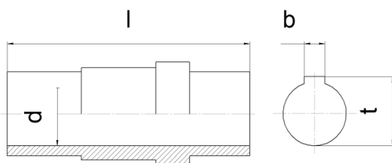
РАЗМЕРЫ ПОЛОГО ВЫХОДНОГО ВАЛА СО ШПОНОЧНЫМ ПАЗОМ KA, KAF, KAZ
