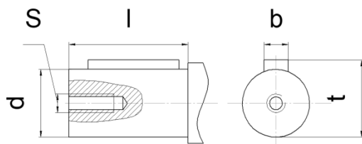
РАЗМЕРЫ ЦИЛИНДРИЧЕСКОГО ВЫХОДНОГО ВАЛА K, KF
