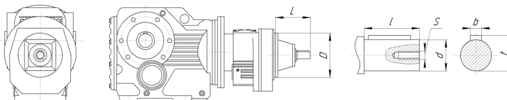
РАЗМЕРЫ ВХОДНОГО АДАПТЕРА ДЛЯ ИСПОЛНЕНИЯ «AD» (ВХОДНОЙ ВАЛ ВМЕСТО ЭЛЕКТРОДВИГАТЕЛЯ)
