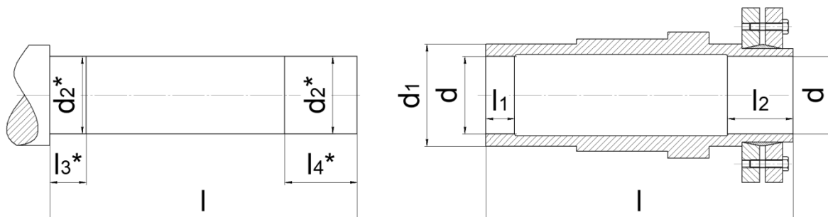
РАЗМЕРЫ ПОЛОГО ГЛАДКОГО ВЫХОДНОГО ВАЛА СО СТЫЖНОЙ МУФТОЙ KH, KHf, KHZ
