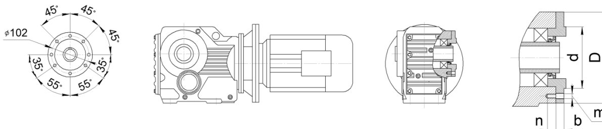
РАЗМЕРЫ ВЫХОДНОГО ФЛАНЦА РЕДУКТОРА KAZ, KVZ
