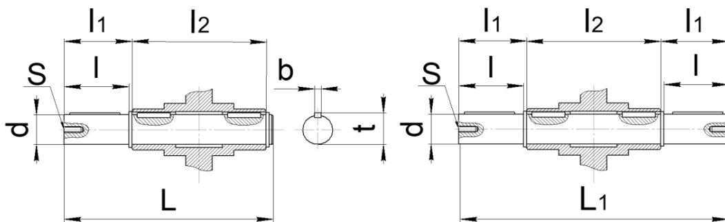
Односторонний выходной вал
