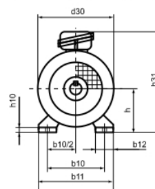
МТН 41, 200–400 (КОНИЧЕСКИЙ ВАЛ)
