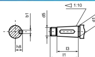
МТН 41, 200–400 (КОНИЧЕСКИЙ ВАЛ)
