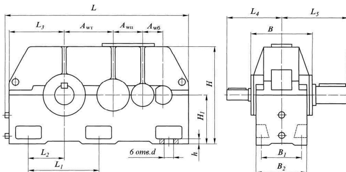
Габаритные и присоединительные размеры редукторов
