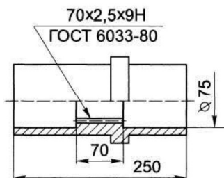
Присоединительные размеры полого вала редуктора 1ЦЗУ-200
