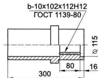
Присоединительные размеры полого вала редуктора 1ЦЗУ-250
